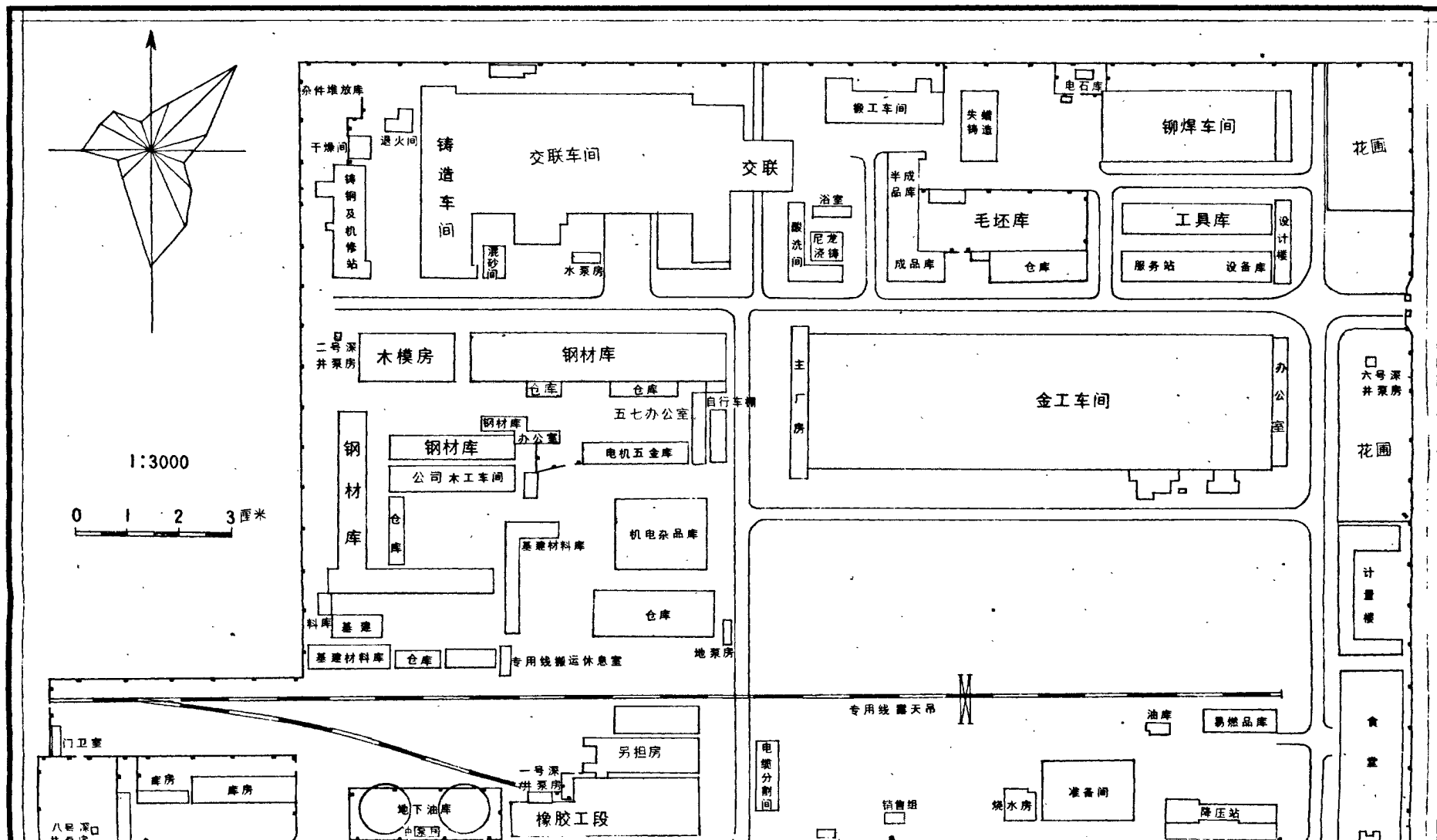
电缆厂厂区总平面图
