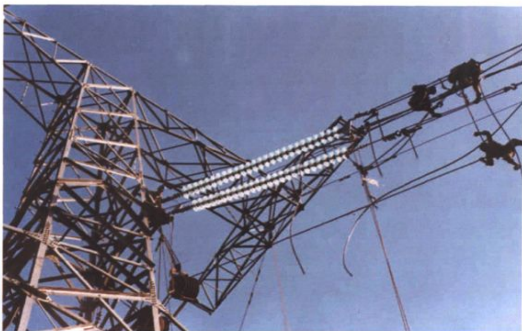
500千伏辽长吉哈佳输电线路耐张塔挂线施工
