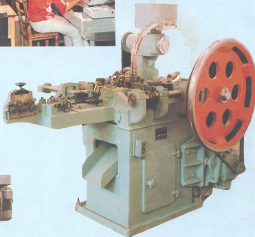
上圖為興寧五金機械廠生產瓦楞釘機 左圖為梅縣市機械廠生產立式破碎機
