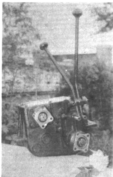
寿光县齿轮箱厂制造的 BJ-212分动器
