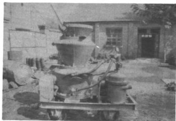
寿光县建筑建材机械厂研制的泰山—75 型混凝土喷射机
