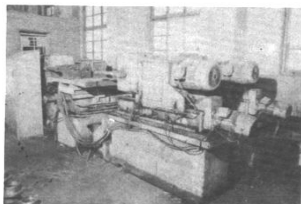
寿光县第二曲轴厂试制成功的495 柴油机双端面三工位组合机床
