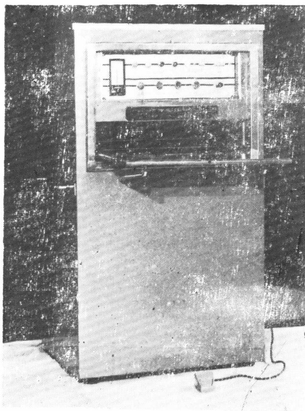
PYL—2型 平型压领机
