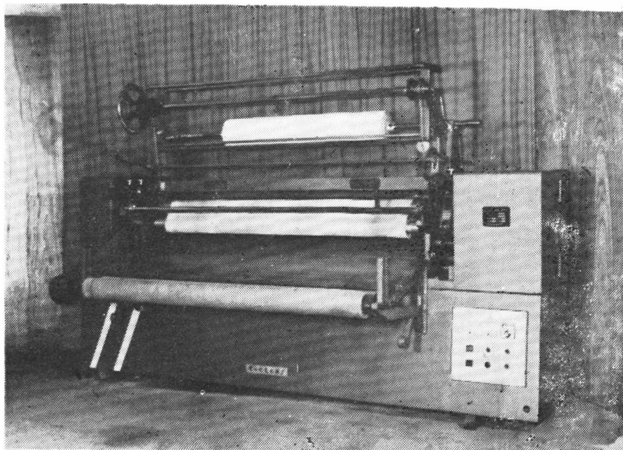
ZJ——215型多功能摺景机
