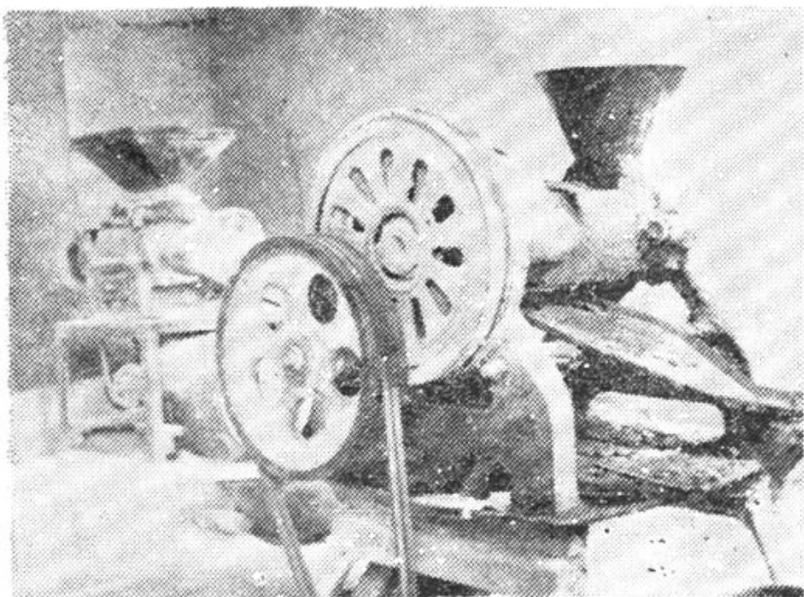
榨油机
