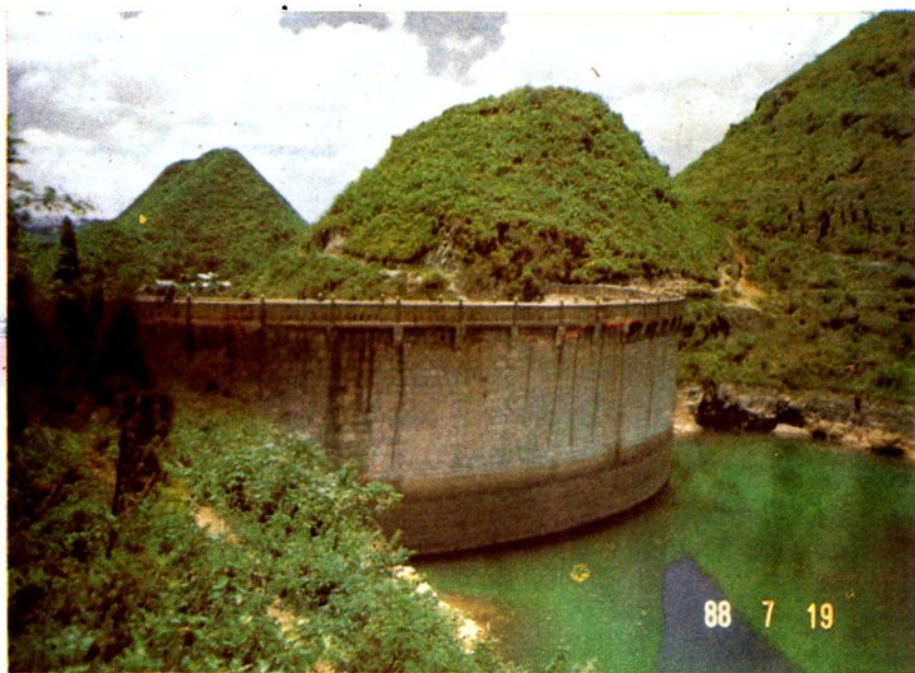
平坝县前进水库
