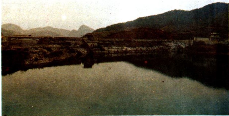
安顺县红岩水库
