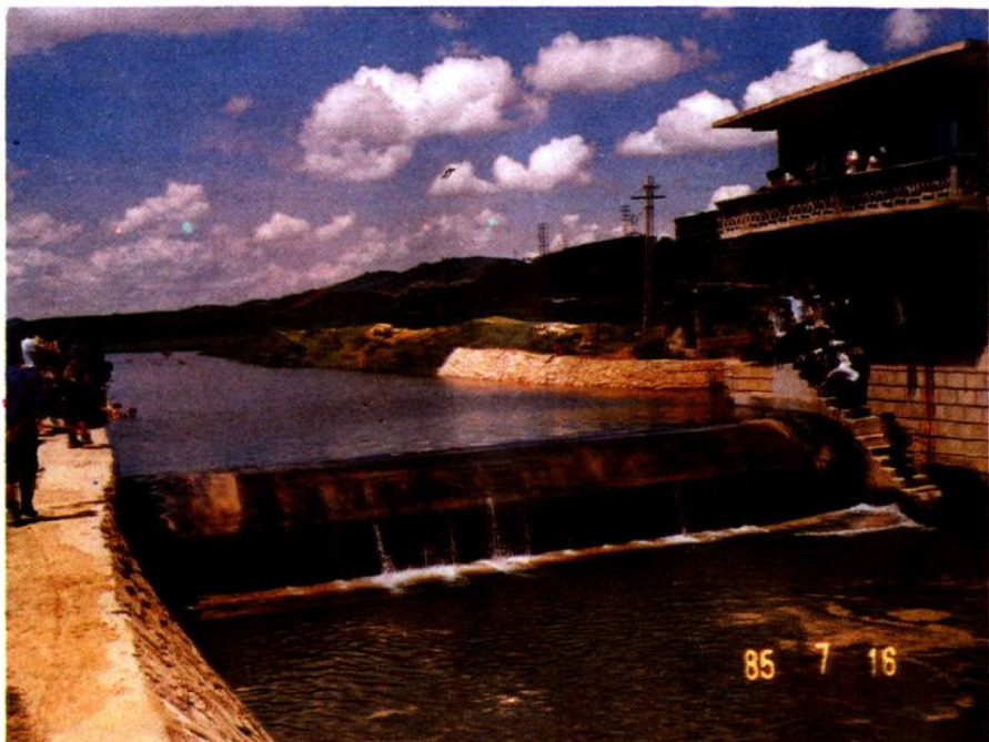
平坝县龙井引水工程橡胶坝
