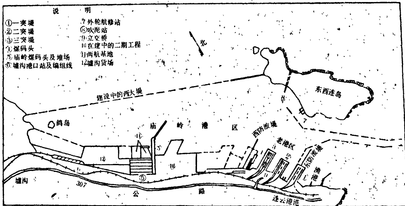
卷首图 连云港港区平面布置示意图
