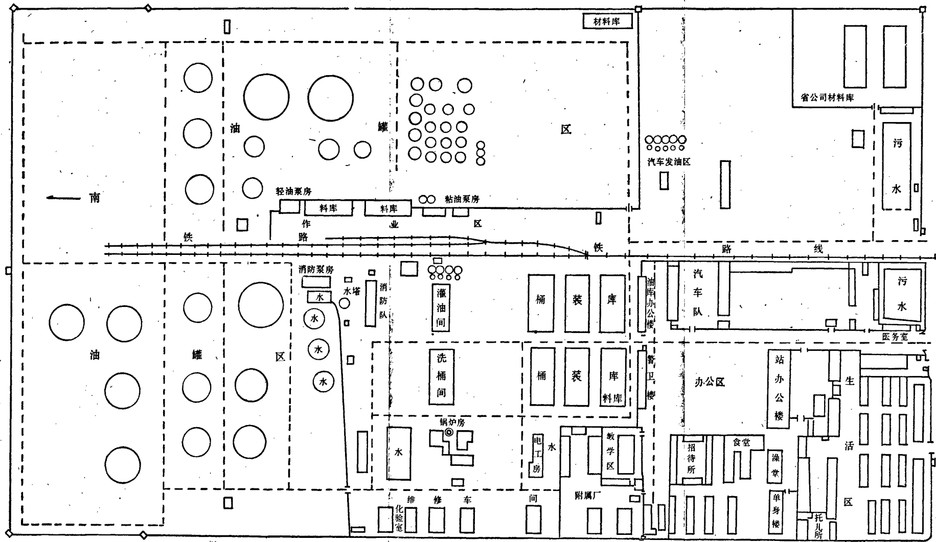
郑州石油站示意图
