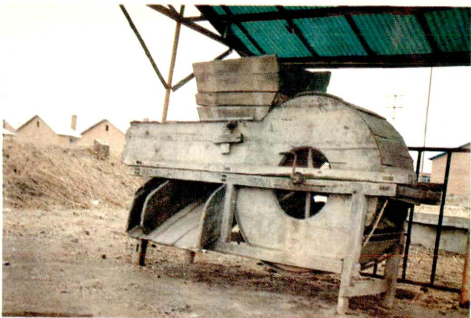
手摇扇车
