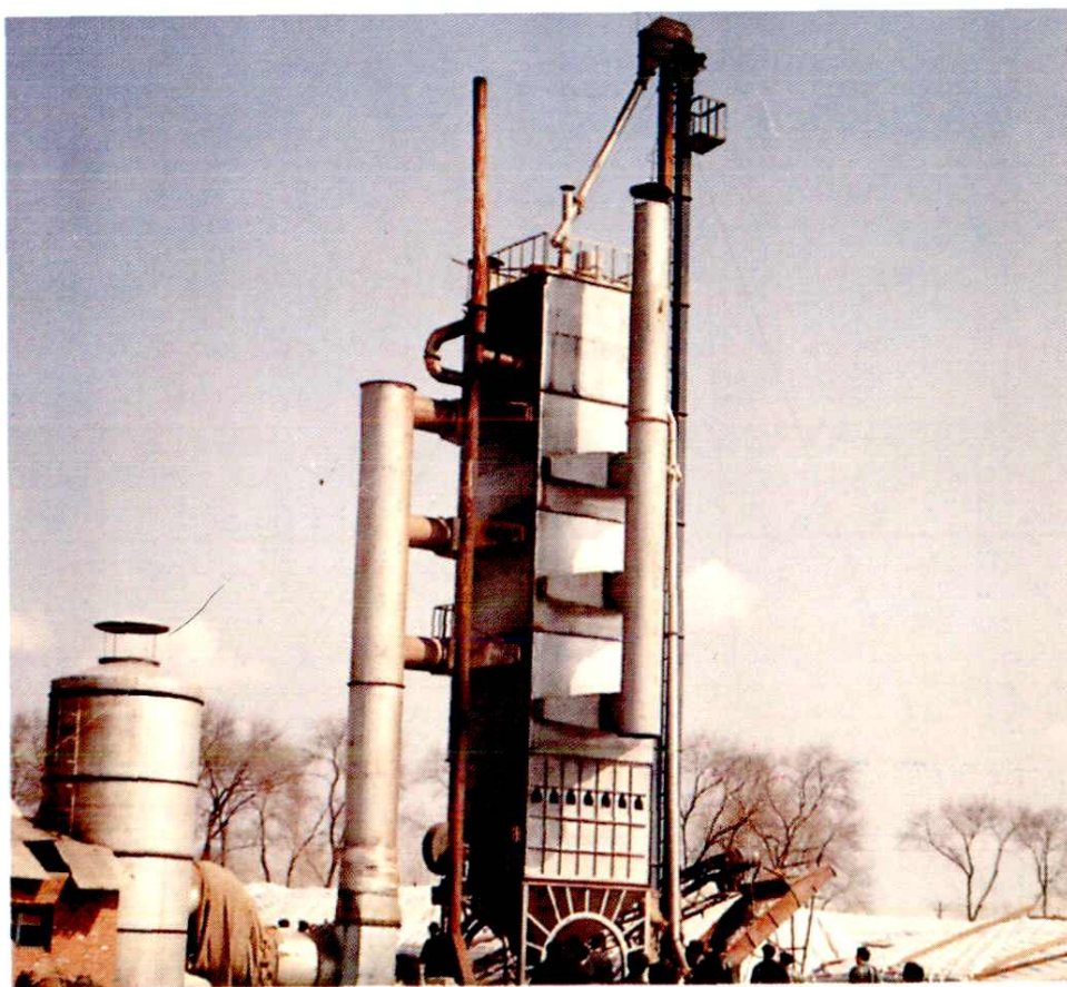
新式烘干塔
