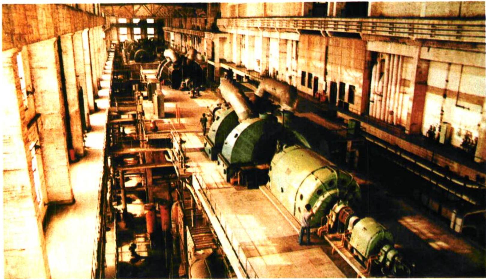
公司安装的永安火电厂 10 万千瓦机组
