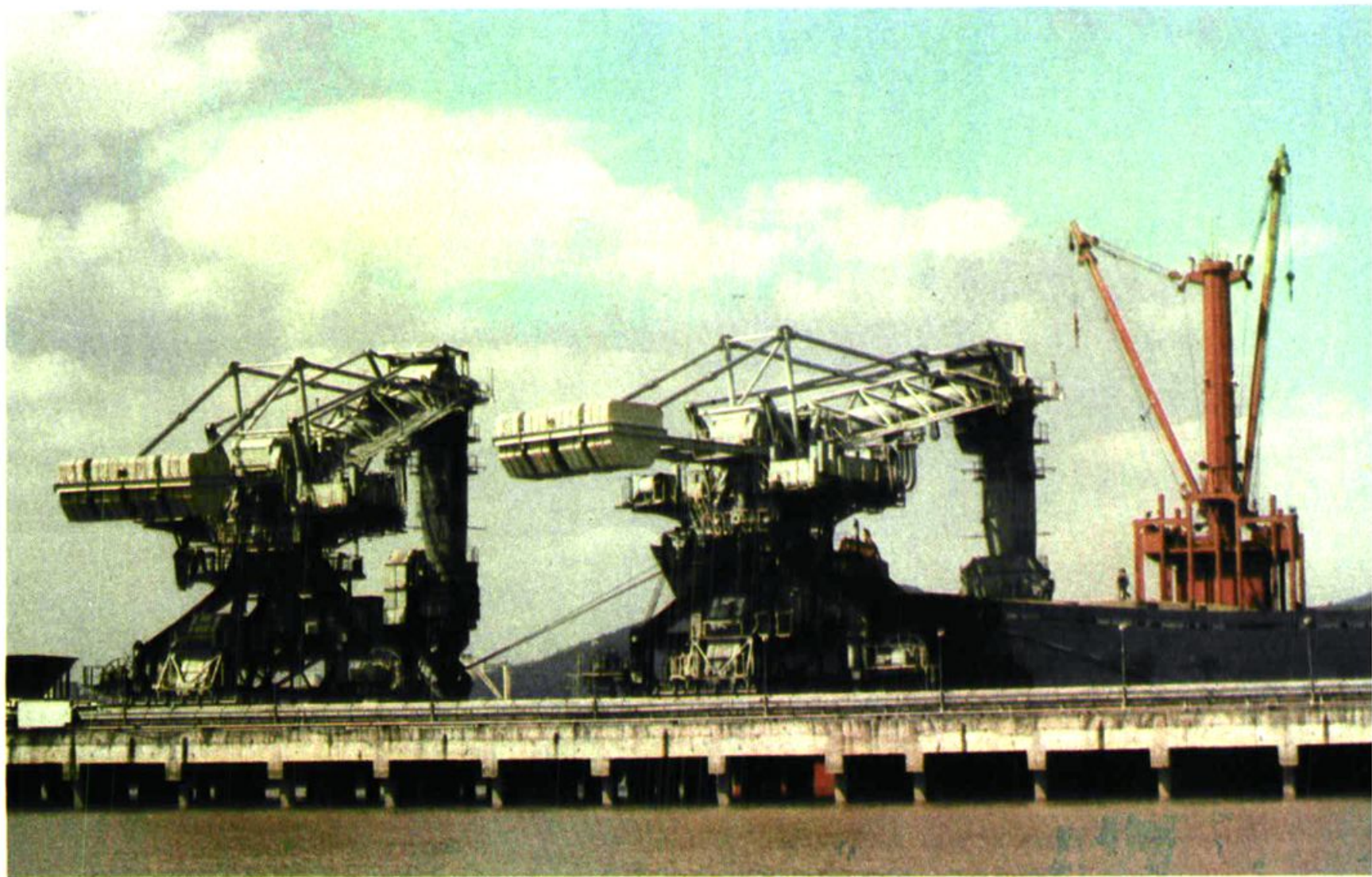
公司安装调试的华能福州电厂大型煤码头卸船机
