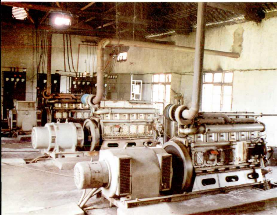
洋峰房水电管理服务公司 480 千瓦发电机组
