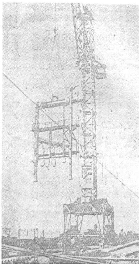
呼和浩特新建热电厂一号锅炉第一片钢架起吊。
