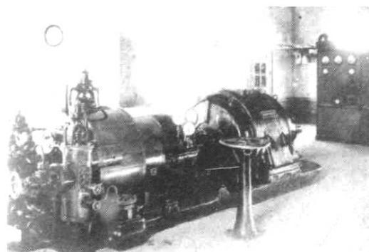
一九二九年——一九四八年老厂 500 千瓦 发电机组，解放战争中已毁。
