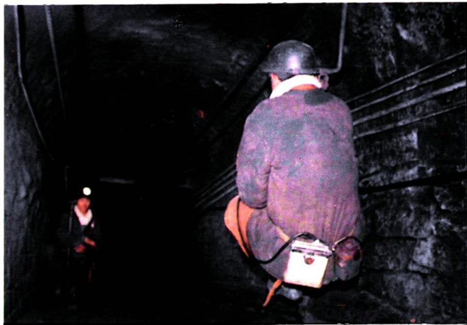
无极绳
