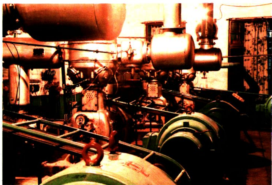
压风机房
