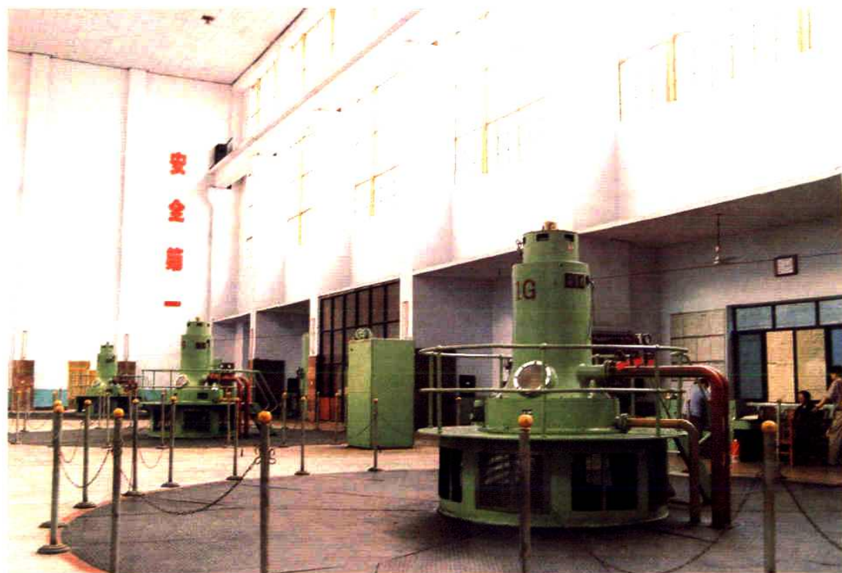
文峰电厂 3 \times 10000 千瓦发电机组
