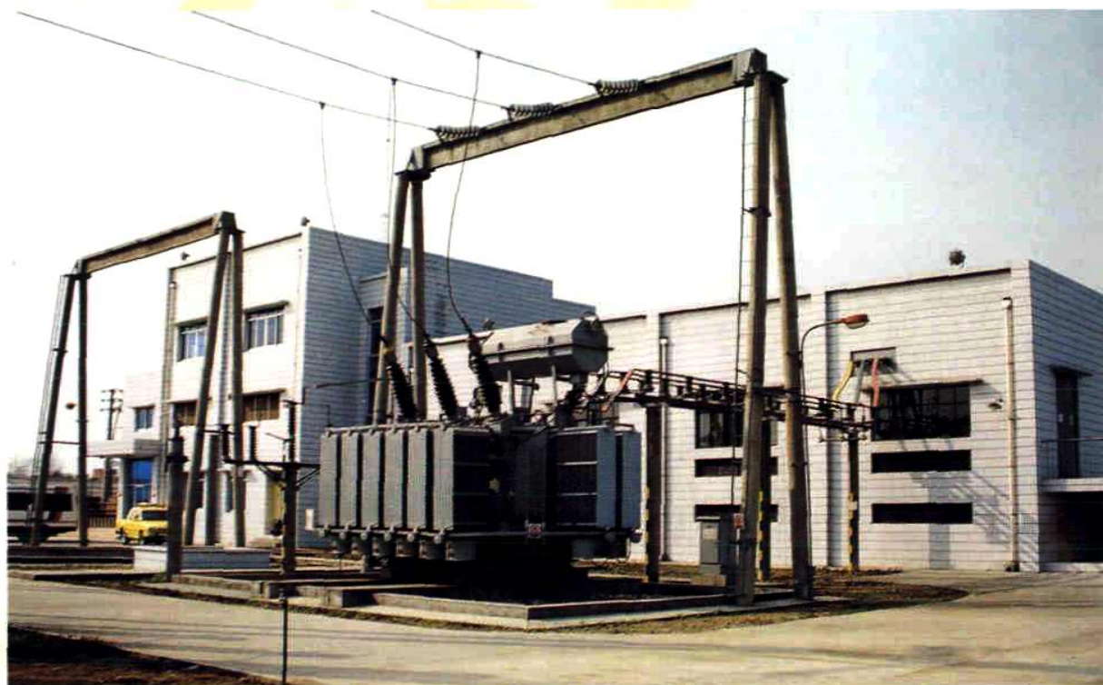
110KV 新皂变电站
