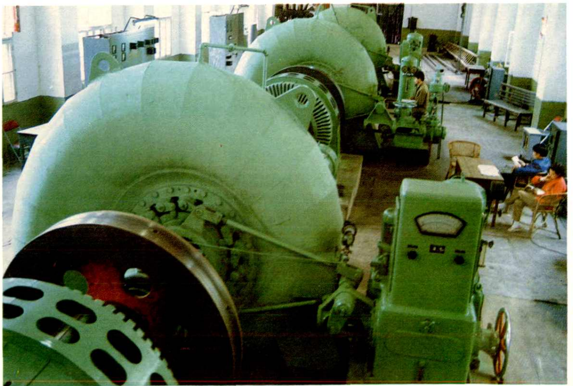
南沙河电站机房
