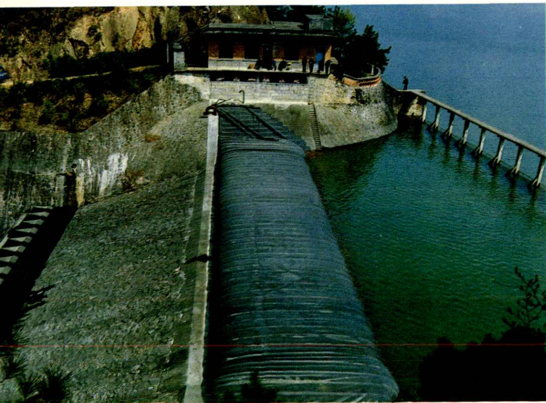
红寺坝水库溢洪道橡胶坝
