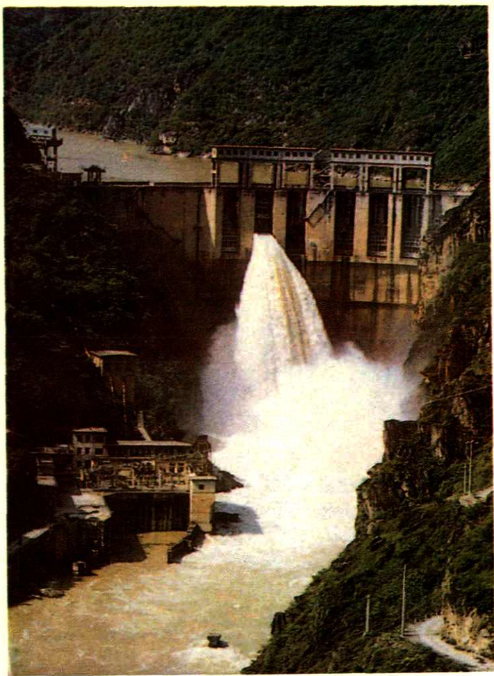
石门水库大孔口泄洪
