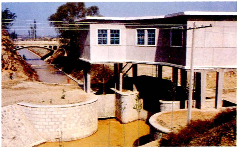
义井分水闸
