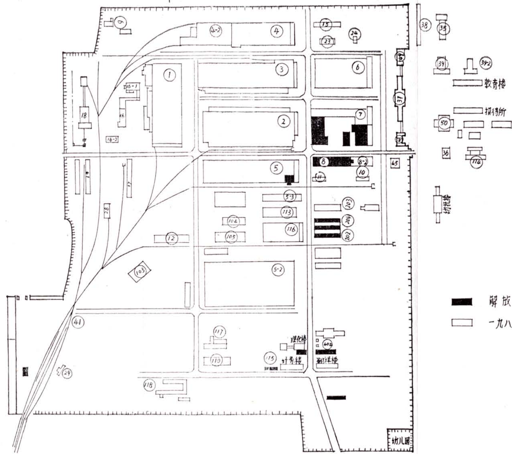
国营晋西机器厂厂区平面图 示意图
