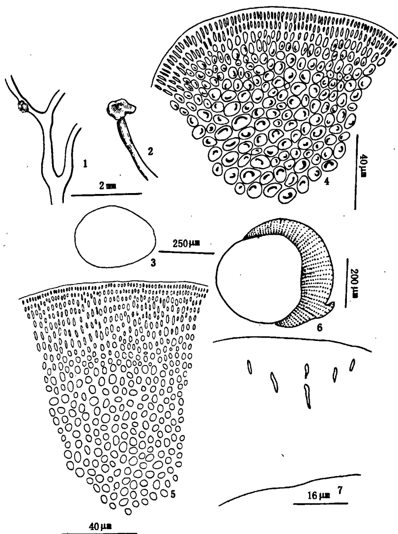
图 1 帚状伊谷藻 Ahnfeltia fastigiata (Post et Ruprecht) Makienko (AST 60-1447) 1. 2. 果孢子体外形图; 3. 中轴横切面观; 4. 5. 部分中轴横切面观; 6. 果孢子体横切面观; 7. 雌性孢子堆中的果胞。
