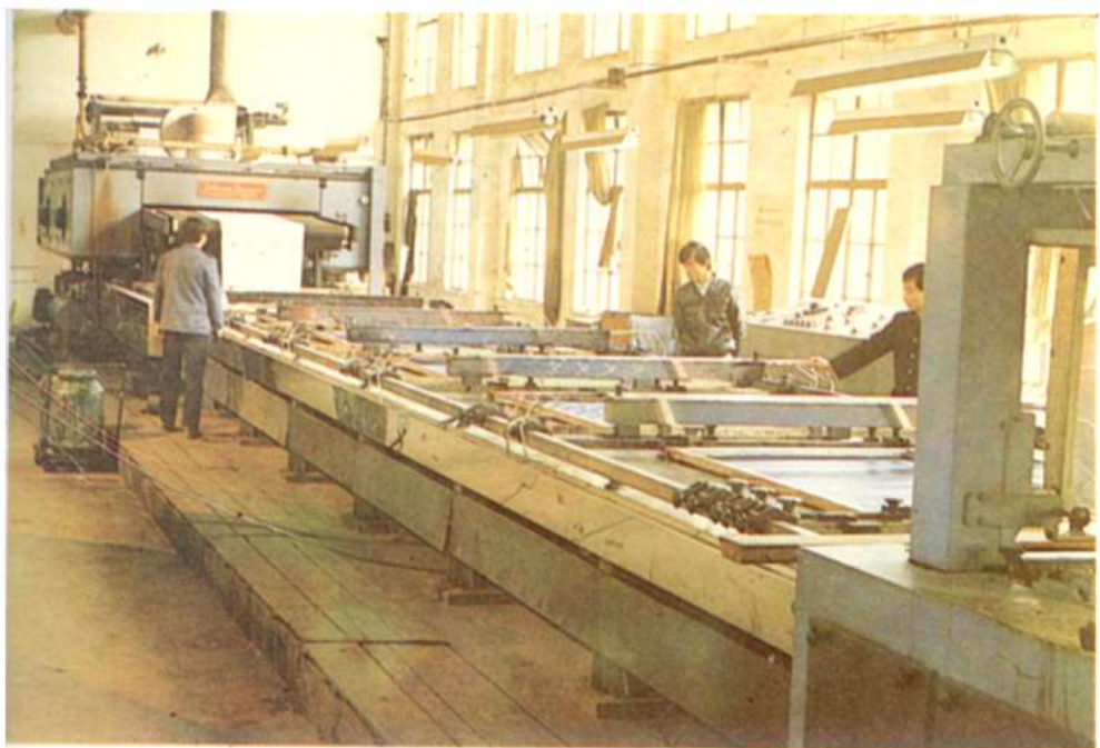
染织厂引进奥地利八色平网印花机
