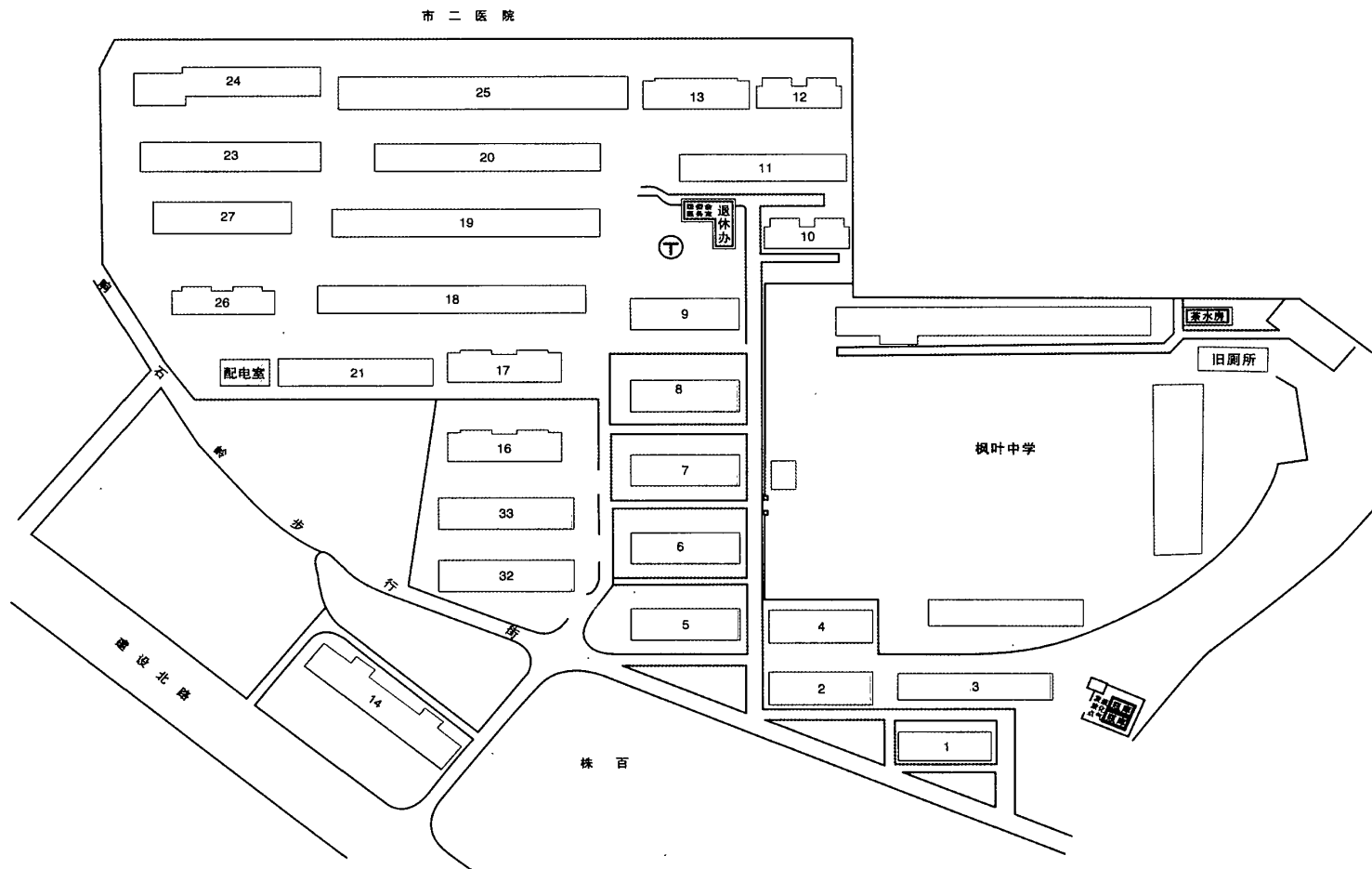
中铁株洲桥梁有限公司第二生活区平面图
