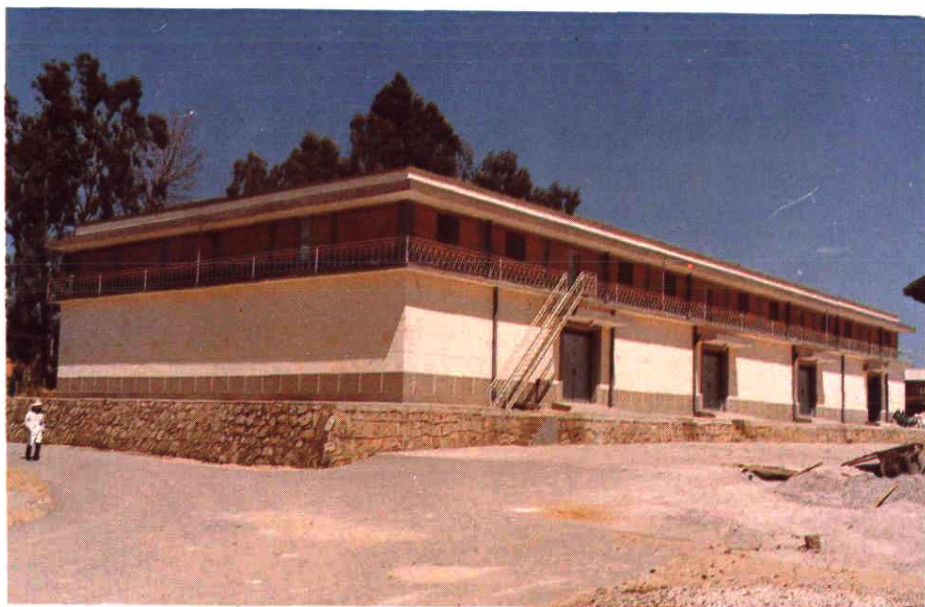
改良苏式仓（安宁县 粮食局直属库）。
