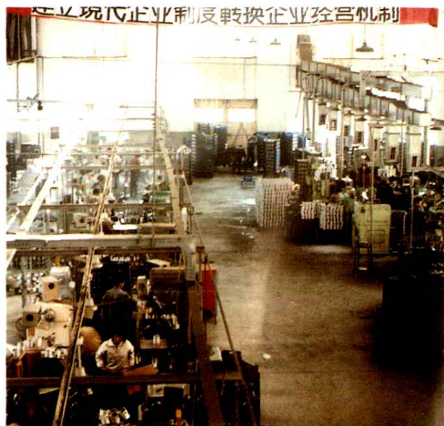
浙江永活股份有限公司活塞装配车间
