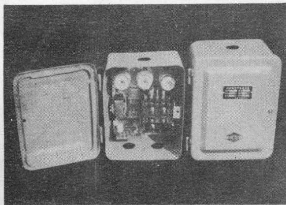
△ 商丘市电器开关厂生产的自动节电 起动器
