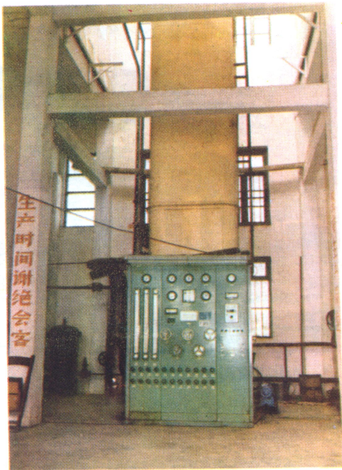
潮州市造船厂的制氧设备
