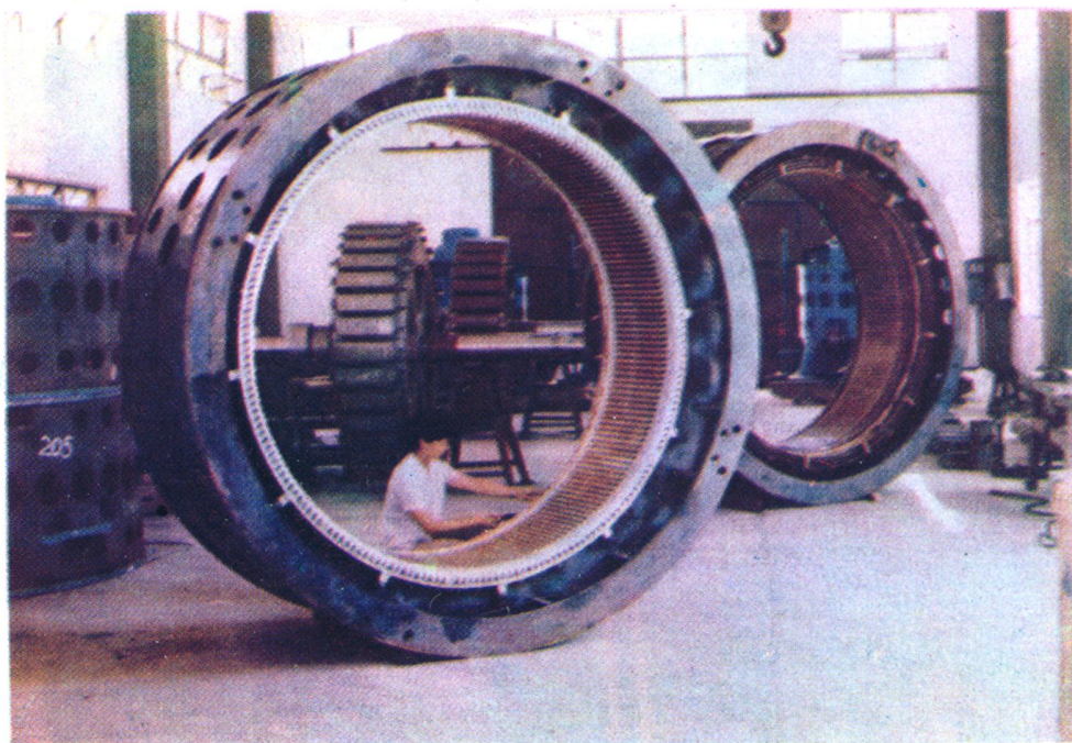
潮州市电机厂生产的韩江牌SF600— 34/2150水轮发电机定子
