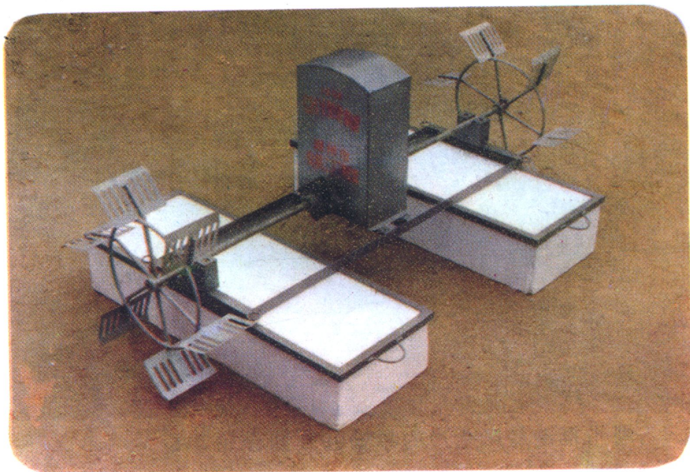
潮州市农机二厂生产的1.5KW水车式增氧机
