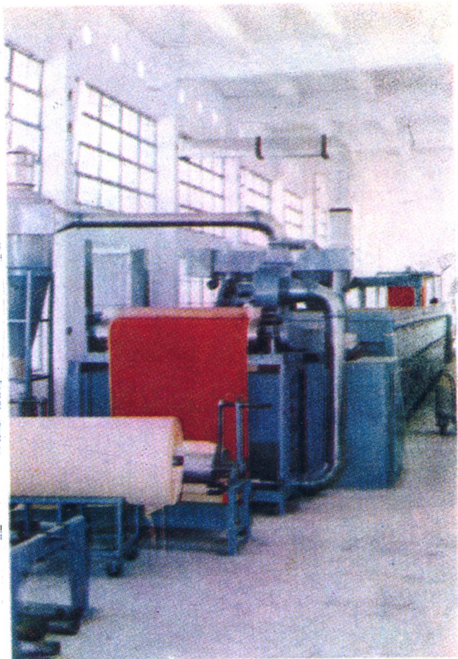
潮州市机械厂、农机一厂制造的DZJ—160 型静电植绒布成套生产设备
