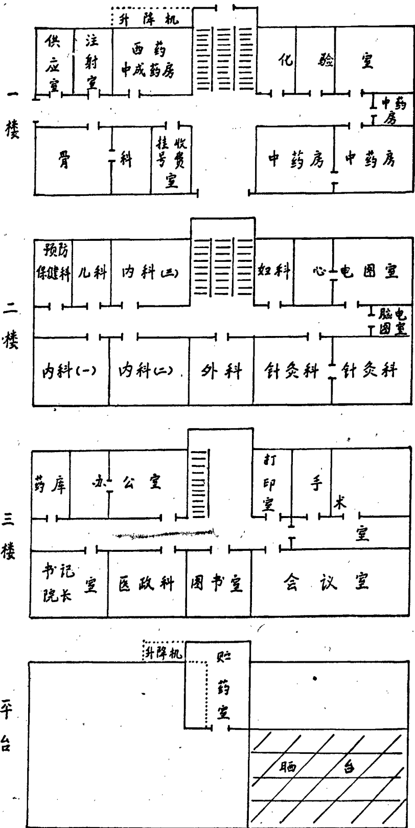
门诊楼分层平面图
