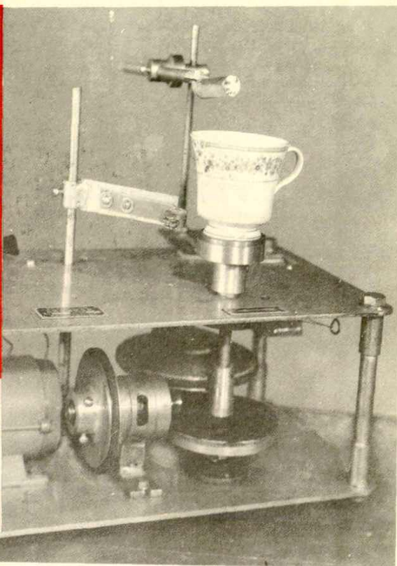
▲ZL104-90 多用无级变速镀金机 (市钟表厂供稿)
