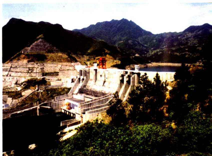
1998年全部建成并网发电的宝珠寺水电站大坝【总装机容量70(4×17.5)万千瓦】
