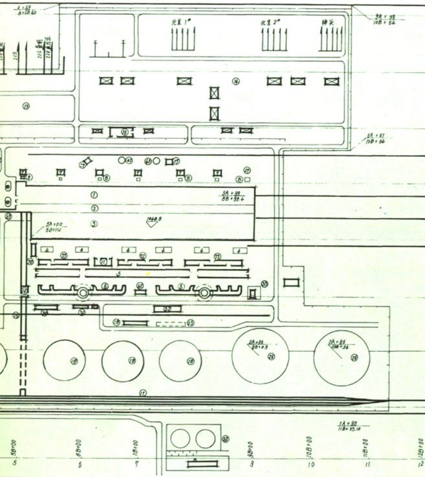
大同发电总厂 总平面示意图
