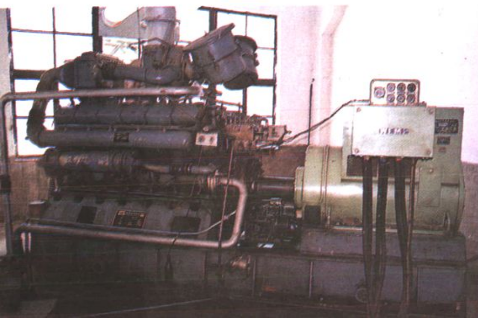
坪上玻璃厂500千瓦发电机组
