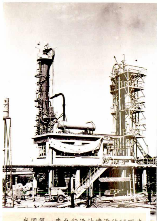
我国第一座自行设计建设的15万吨原油常减压蒸馏装置,在上海炼油厂建成(1956年)
