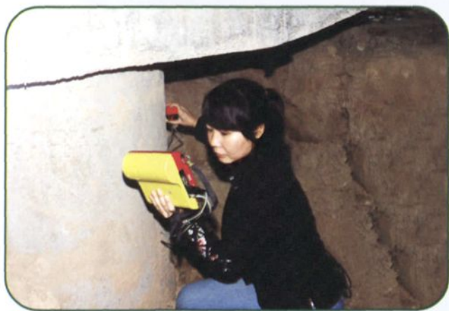
检查组技术人员用仪器检测桥梁混凝土保护层厚度（左图）和强度（右图）
