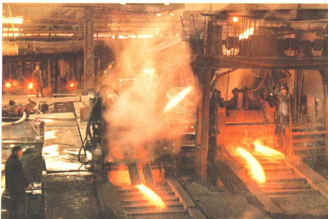
→ 开坯轧机正在进行热轧
