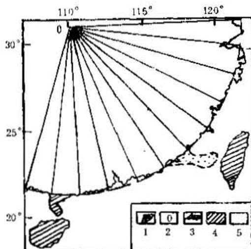
图 2-1 华南弧形海岸
