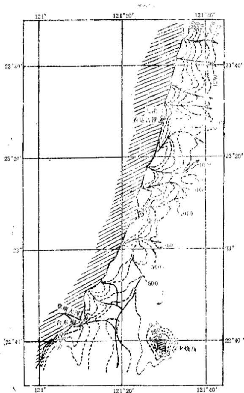
图 2-4 台东海岸山脉岸外溺谷图
