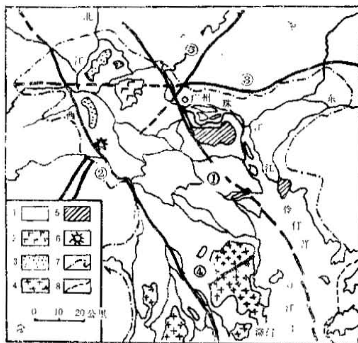
图 2-3 珠江三角洲西、北江部分主要断裂系统图
