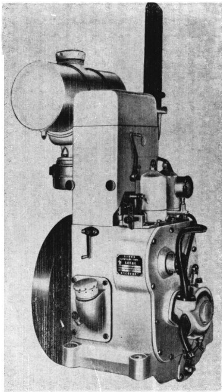
1105 型柴油机
