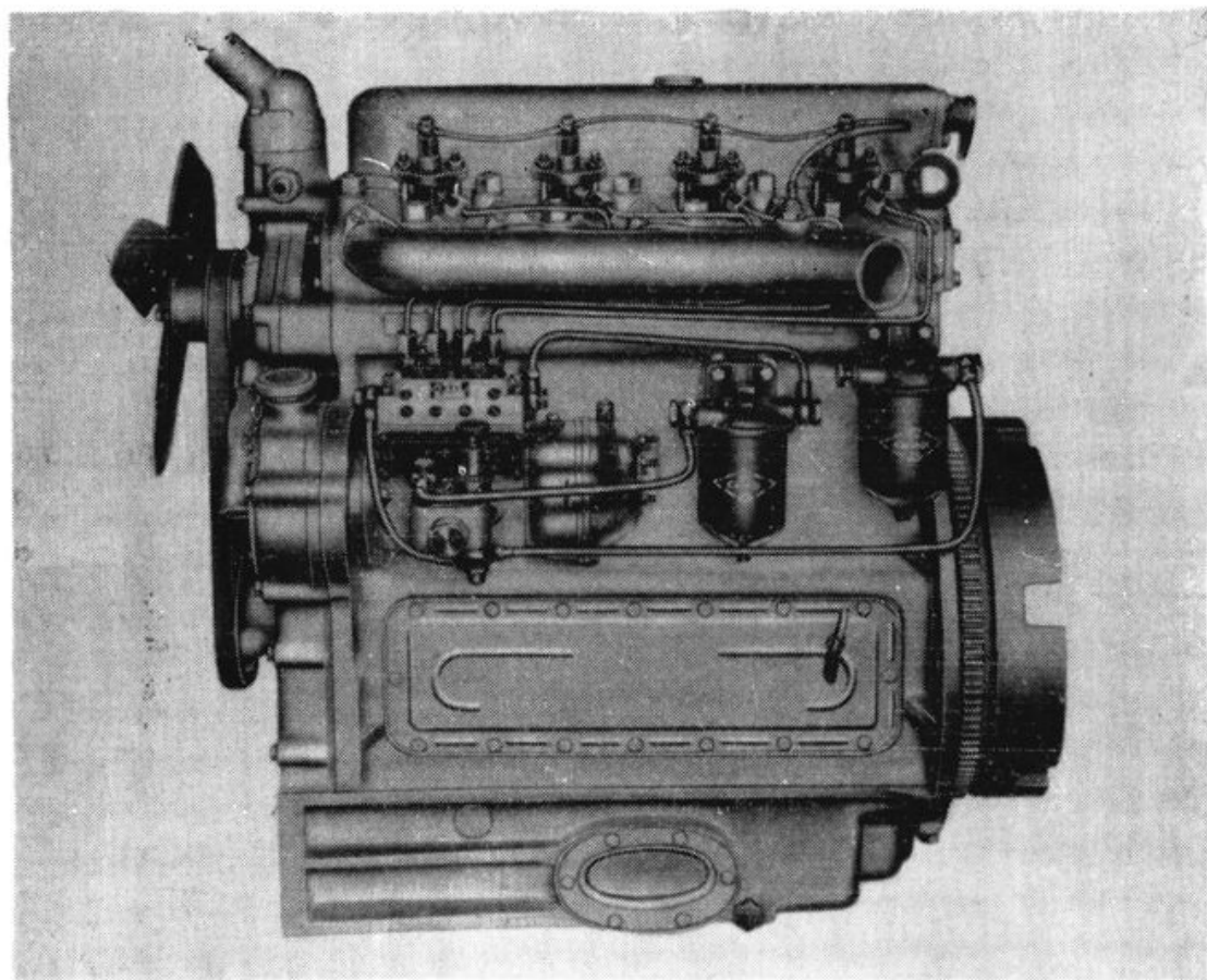
495 型 柴 油 机
