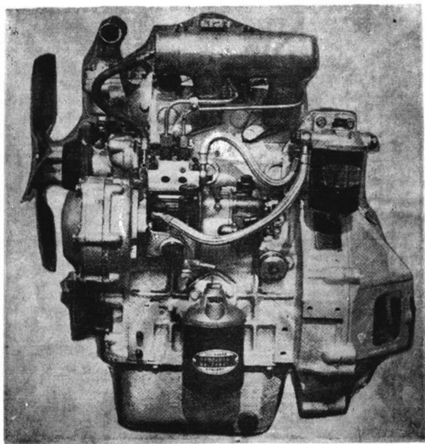
2 9 0 Q型柴油机
