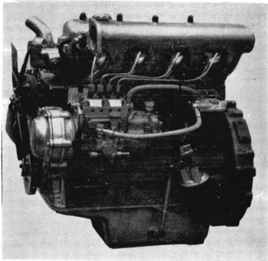
4 9 0 Q型柴油机
