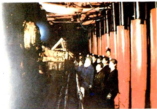
我国自己设计制造的第一套原煤层综采机组正在采煤。
