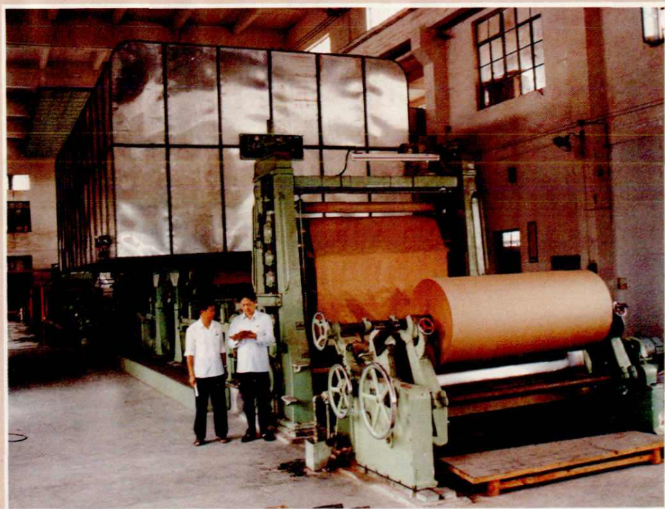
图为纸厂1988年投产的新型长网多缸薄页纸机在进行生产。
