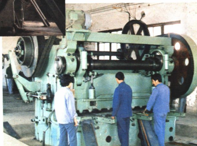
◁ \phi 2.2 \times 6.5m 水泥大磨
