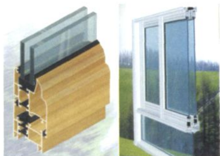
隔热型装饰铝合金型材
