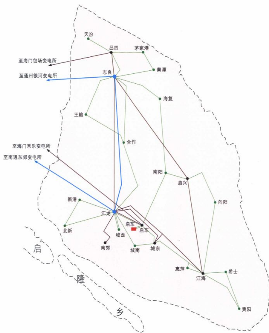
2005年底启东电网地理接线示意图
