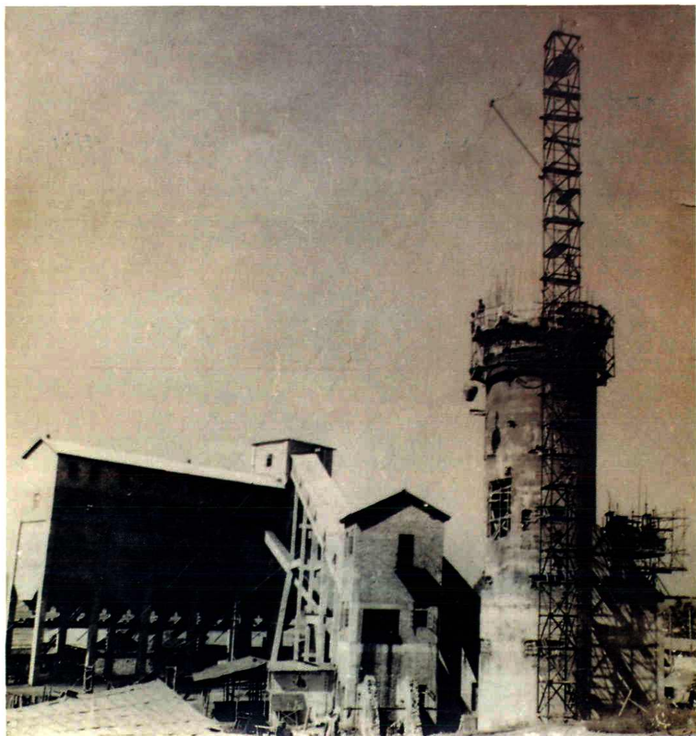
合山矿务局石村立井钢 筋混凝土井架滑模施工
