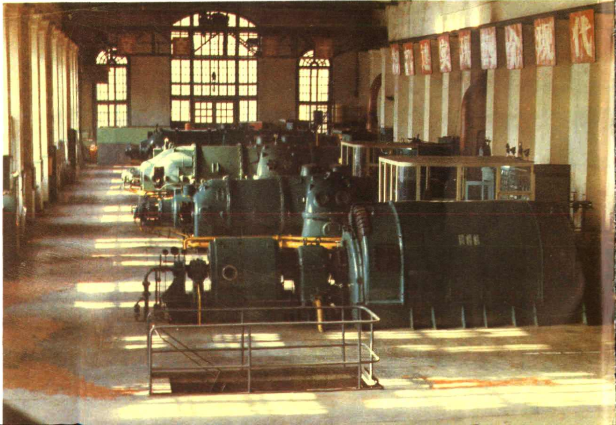
哈尔滨发电厂30年代幅流式汽轮发电机
