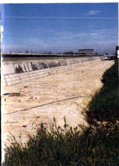
沿海标准堤塘
