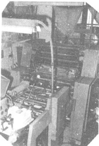
江津县印刷厂胶印机
