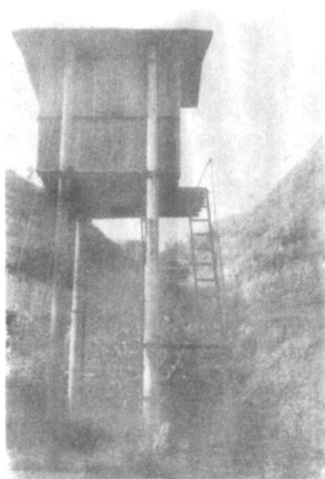
建个线路末杆（个旧507）P1351 舒予明 摄
