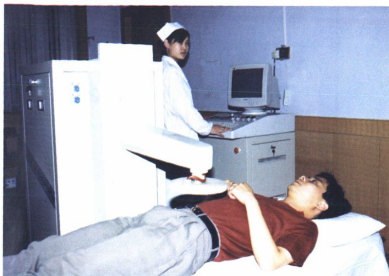
HG-2000 体外高频热疗机
