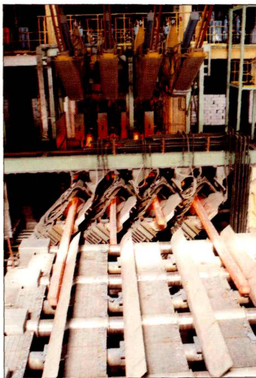
3号连铸机
