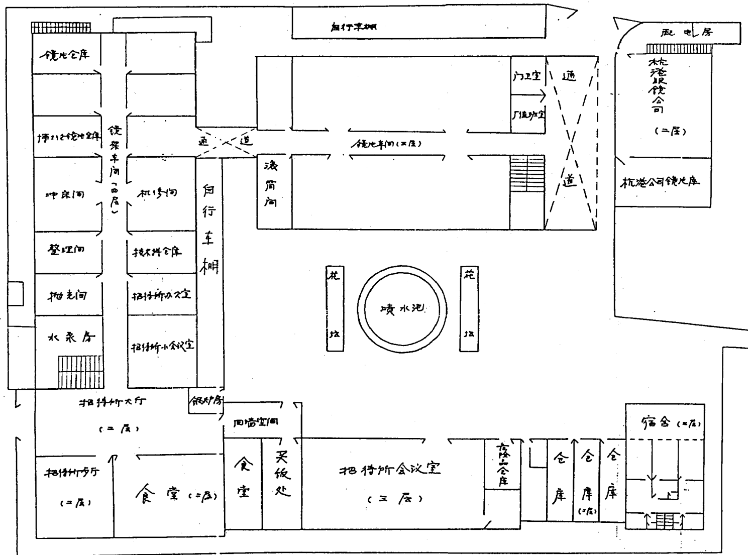
杭州毛源昌眼镜厂平面图
