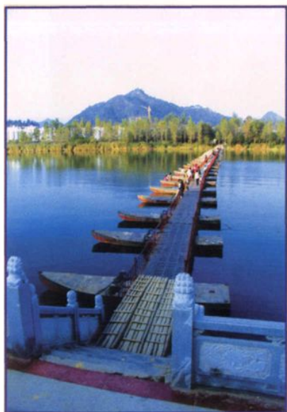
马家洲浮桥
