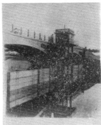
黑河坡张拦河多铰式自动翻转闸
